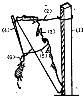
图3 石压法 (1) 木桩 (2) 拉绳 (3) 石块 (4) 铁针 (5) 饵绳 (6) 饵食
