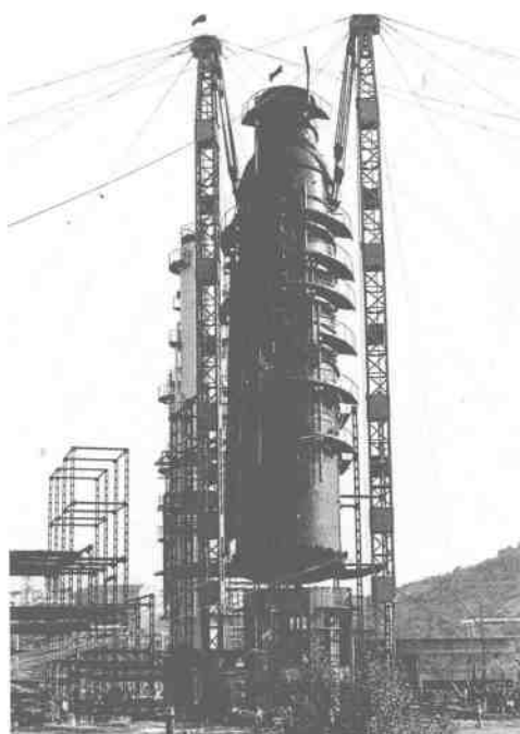
吊装常减压装置蒸馏塔
