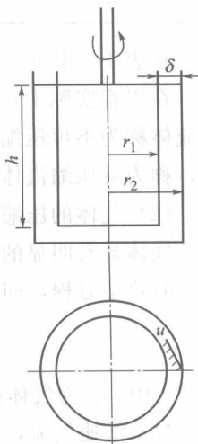
图 1-4 旋转黏度计
