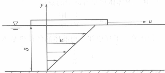
图 1-3 速度分布
