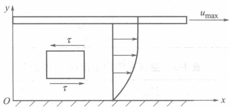
图 1-2 牛顿平板实验速度、切应力分布
