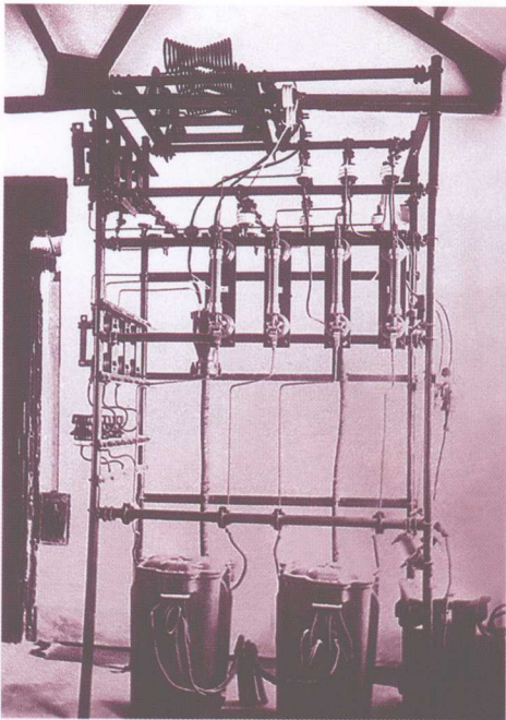
南满洲电气株式会社时期，地区 3.3 千伏变电设备
