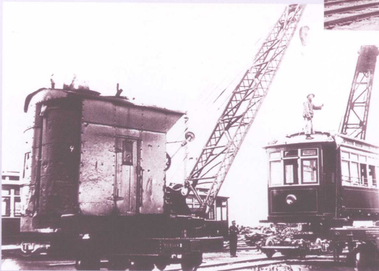
南满洲铁道株式会社时期，有轨电车吊装作业
