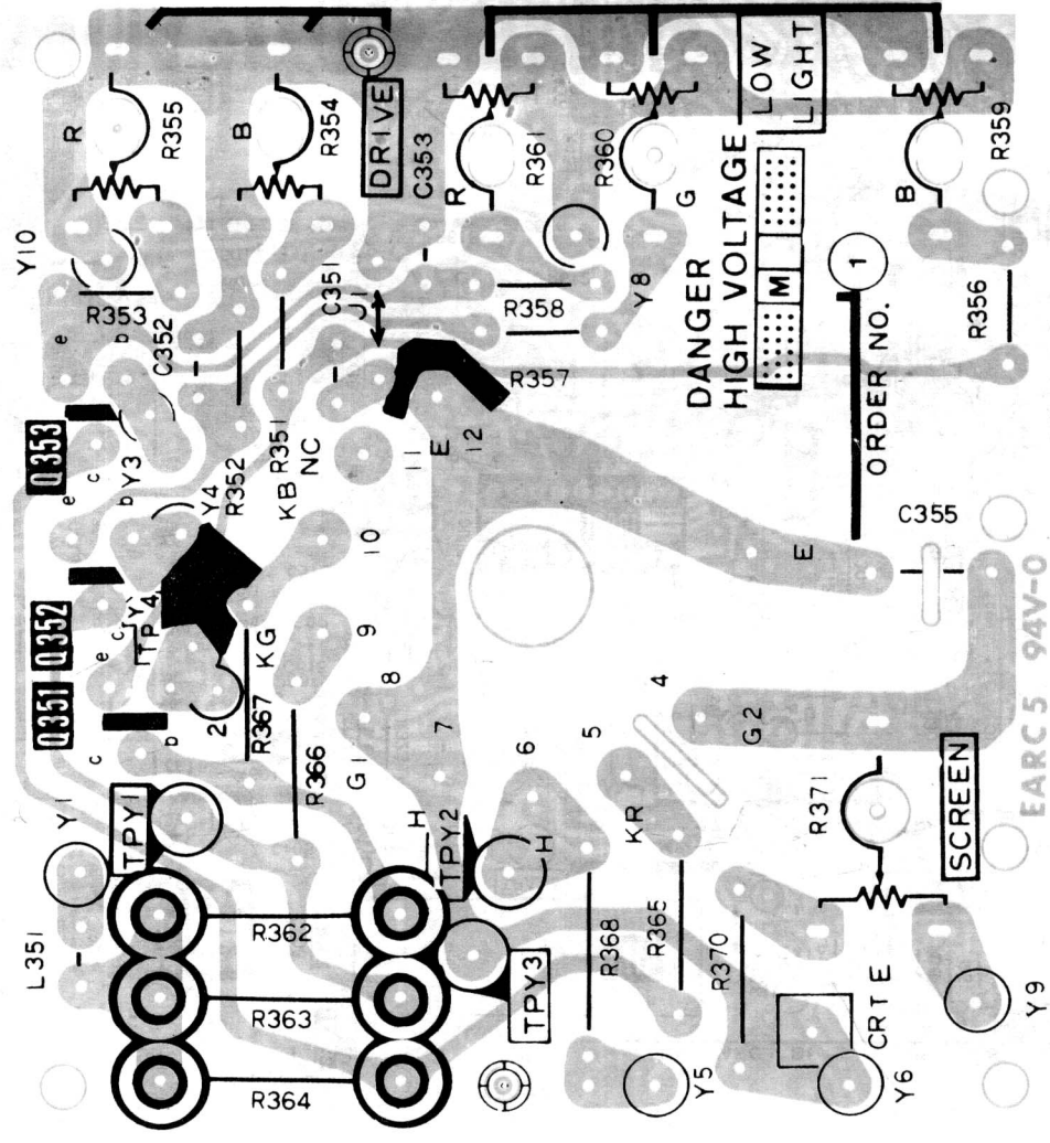
显像管电路板
