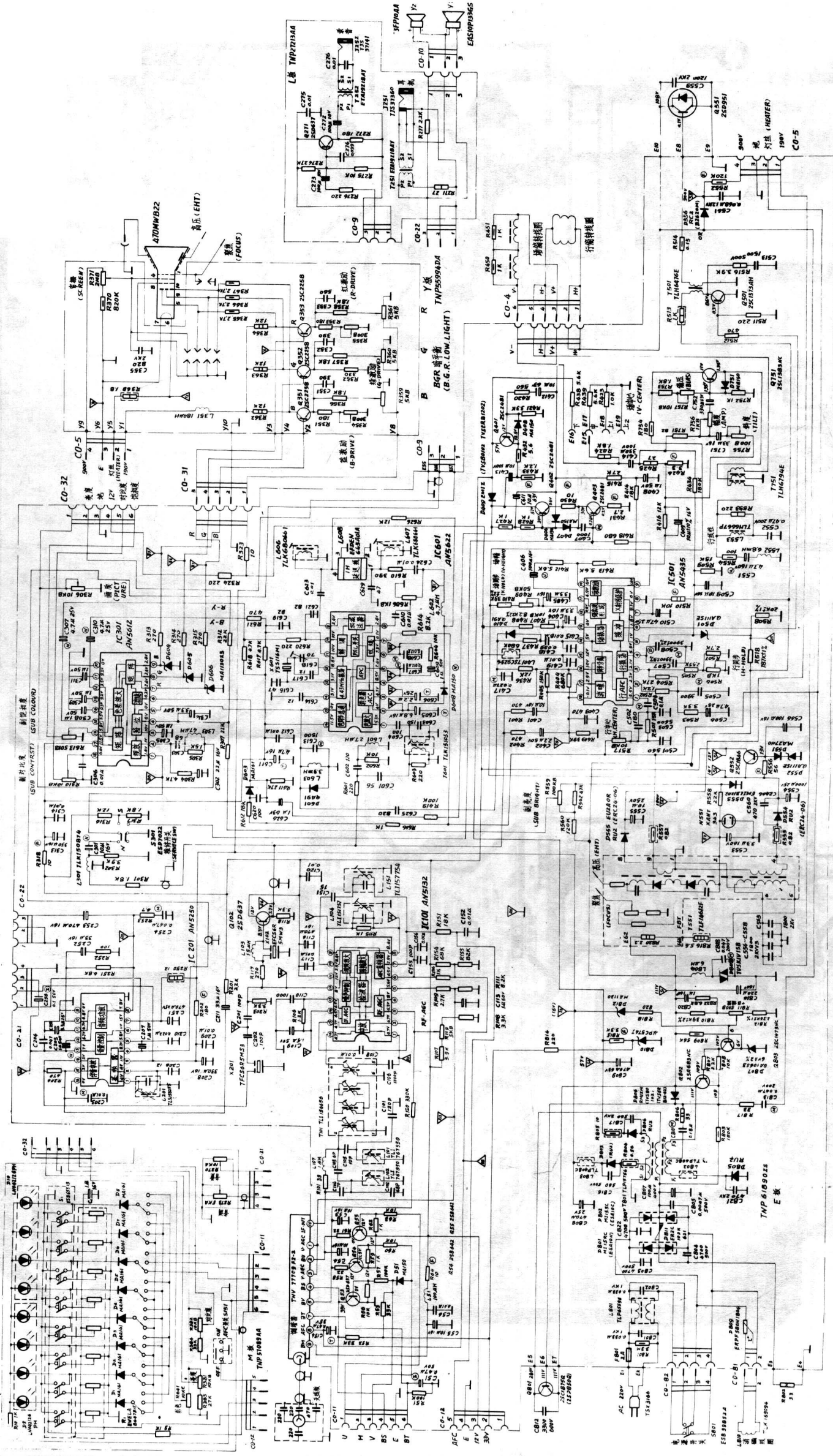
长虹牌CJ47A型彩色电视机电路原理图
