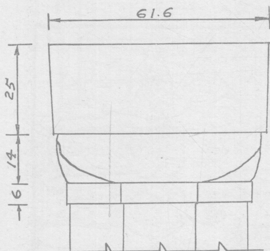
III, 第001號 柱頭特寫
