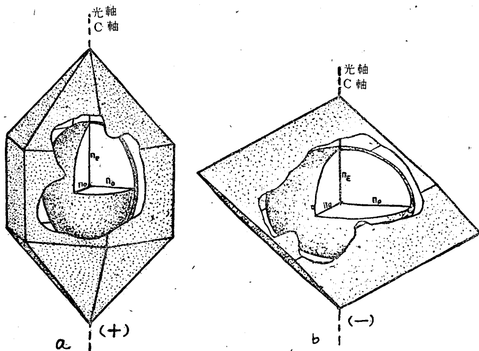
图 296 一轴晶光率体
