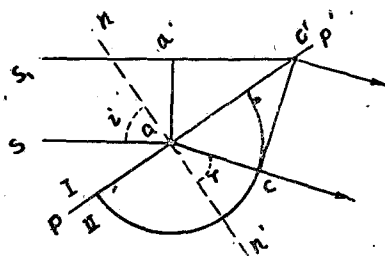
图 291 光的折射
