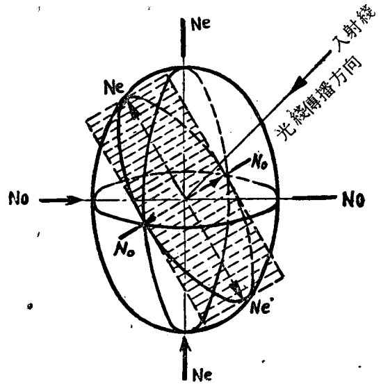
图 297 根据光率体确定光在晶体中的振动方向和相应的折光率
