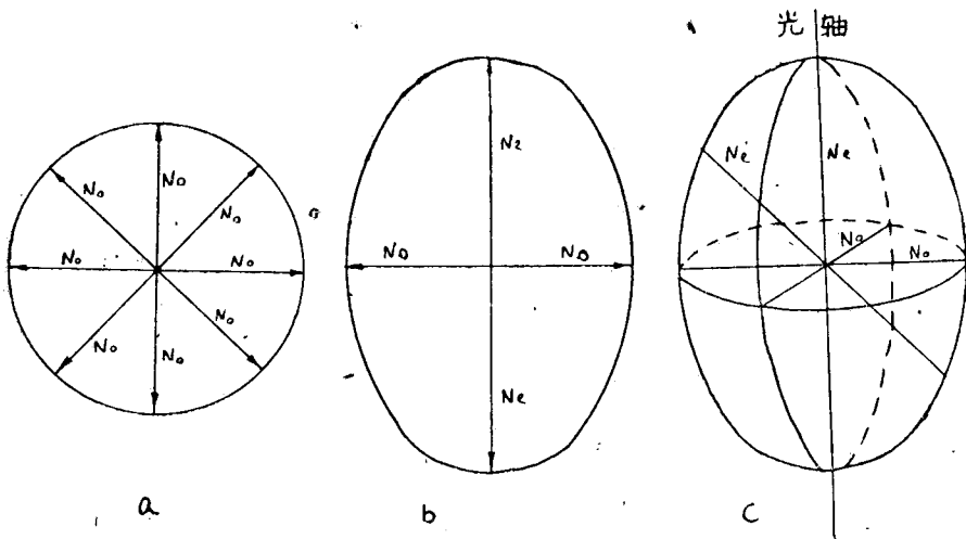
图 295 一轴晶光率体的作图
