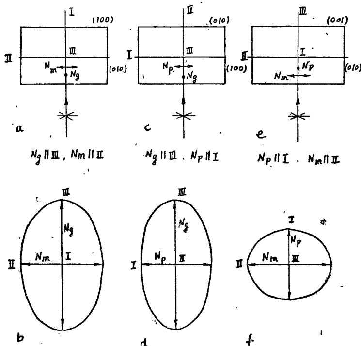
图 298 二轴晶光率体的作图
