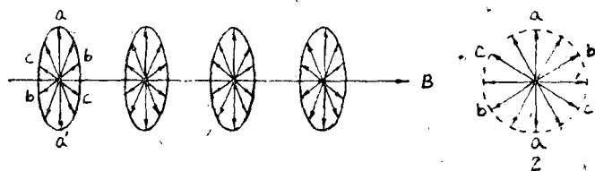
图 288 自然光
