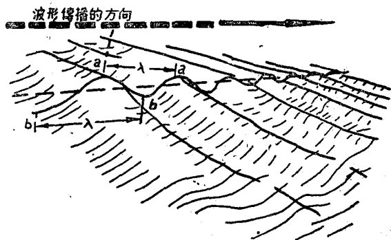
图 286 水波
