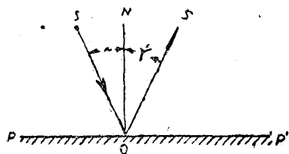
图 290 光的反射
