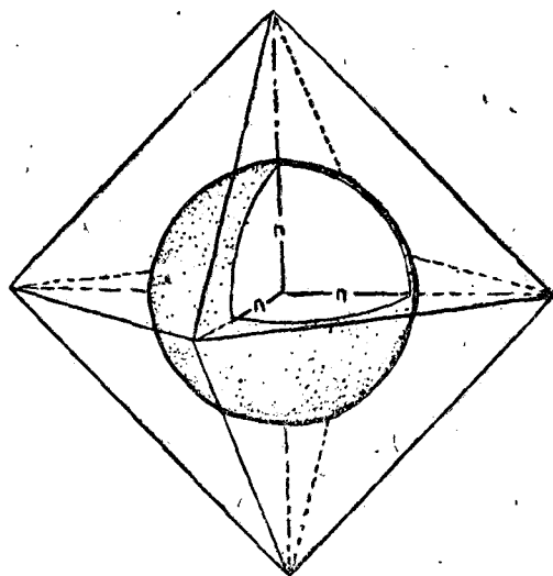
图 293 均质体的光率体
