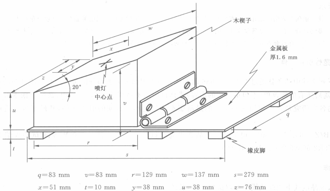
图 1 喷灯底座固定用楔子
