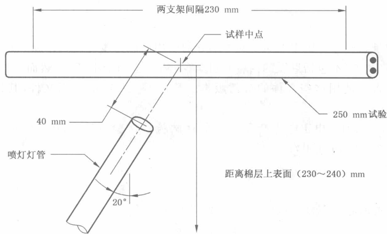
图 1 试样及喷灯位置示意图
