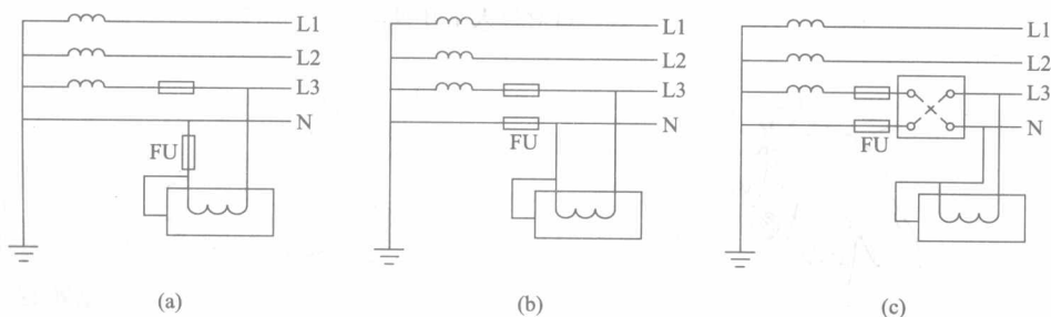
图 1-12 单相电器保护接零的错误接法
