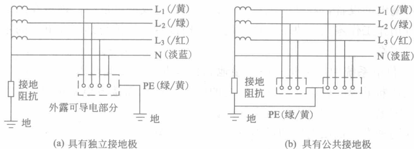
图 1-9 低压电网 IT 系统接线方式
