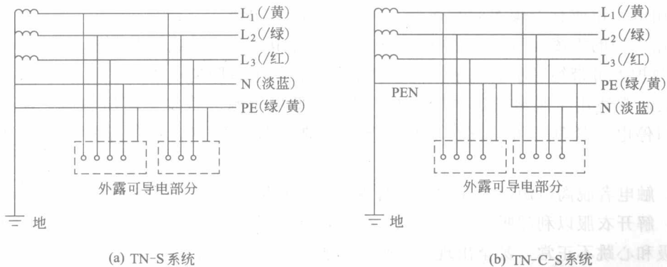
图 1-7 低压电网 TN 系统接线方式
