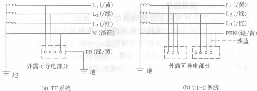
图 1-8 低压电网 TT 系统接线方式
