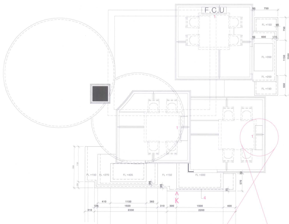
池塘局部J平面图
