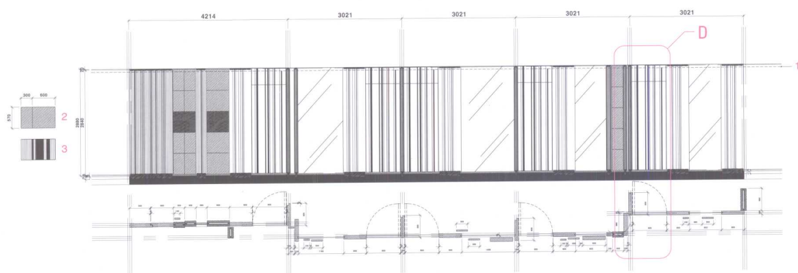
大厅立面图A
