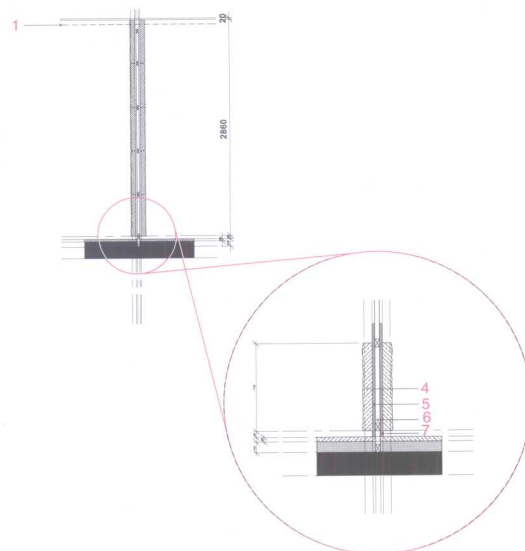
艺术墙剖面图H
