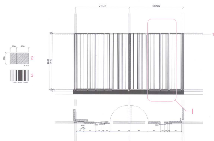
大厅立面图G
