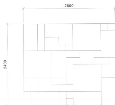
地板拼花详图
