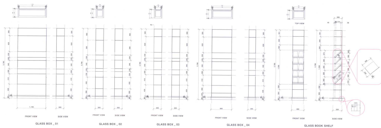
入口大厅玻璃盒子剖面图E
