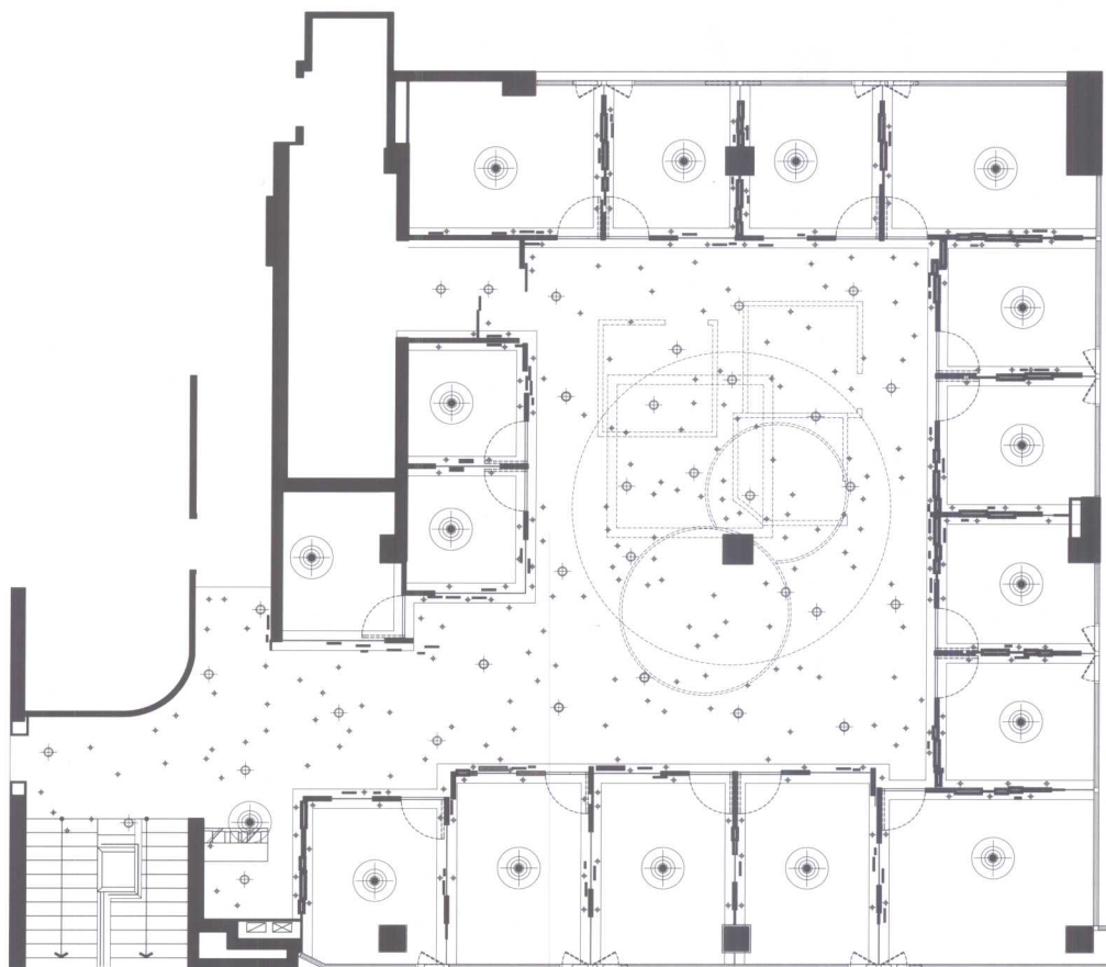
天花平面图
