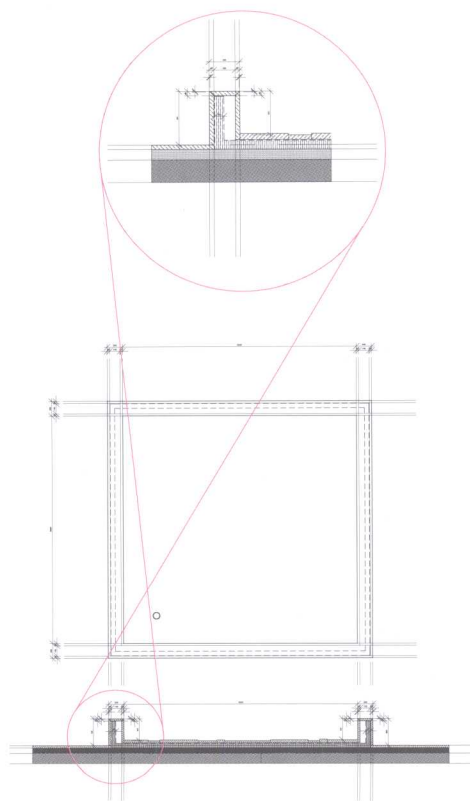
池塘剖面图
