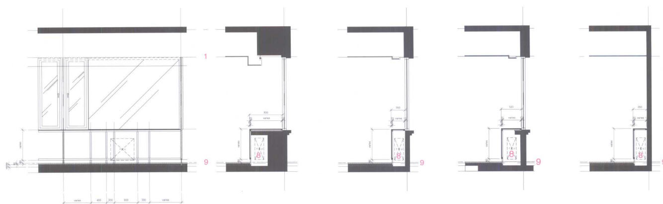
F.C.U 墙剖面图
