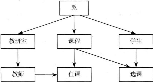
图 1-4 网状模型示意图
