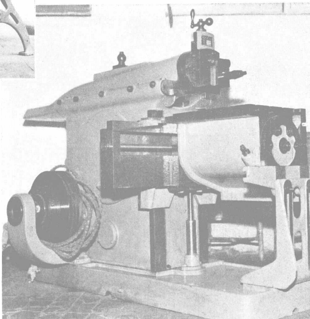
苏州铁工厂产品之一——牛头刨床
