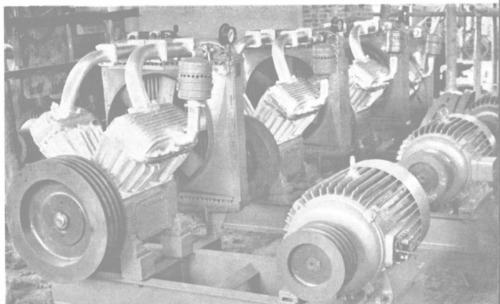
苏州化工机器厂产品之一——空气压缩机
