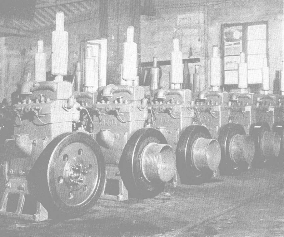
苏州动力机器厂产品之一——内燃机
