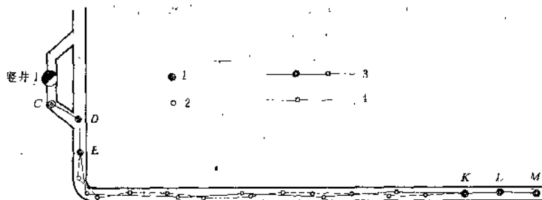
图 2-1 井下经纬仪导线敷设示意图
