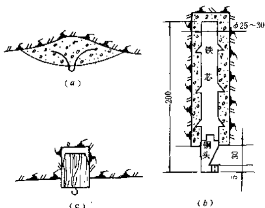
图 2-2 导线点构造图 单位: mm
