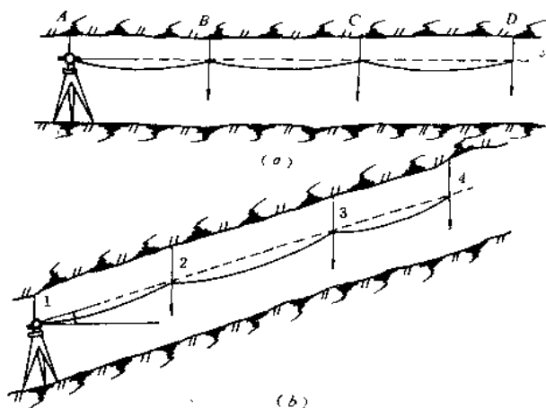
图 2-3 导线边丈量
