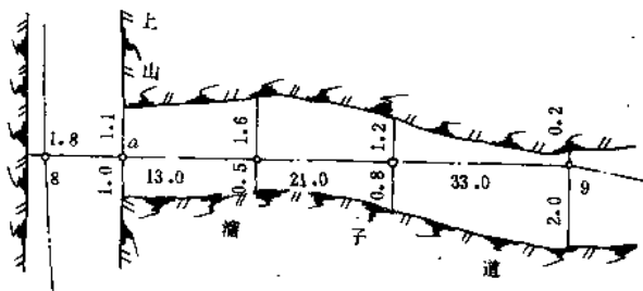
图 2-4 碎部测量草图
