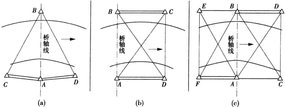
图 9-1 三角控制网
