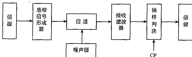
图 1-4 数字基带传输系统模型
