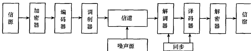
图 1-3 数字频带通信系统模型
