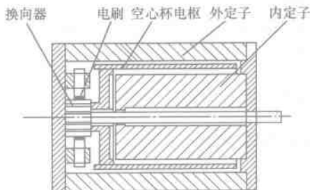
图 1-2 空心杯电枢永磁式直流伺服电动机结构简图
