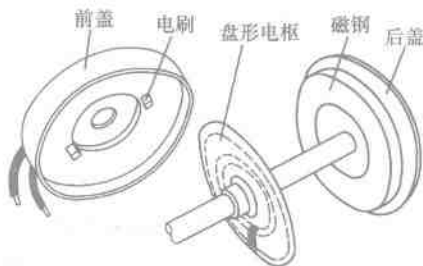
图 1-1 盘形永磁直流伺服电动机结构示意图
