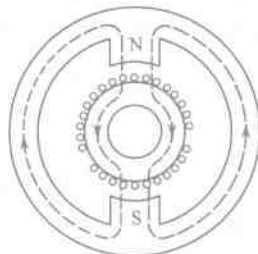
图 1-3 无槽电枢直流伺服电动机结构简图
