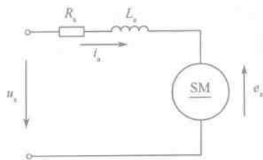
图1-7 直流伺服电动机的等效电路 直流伺服电动机的等效电路如图1-7所示。
