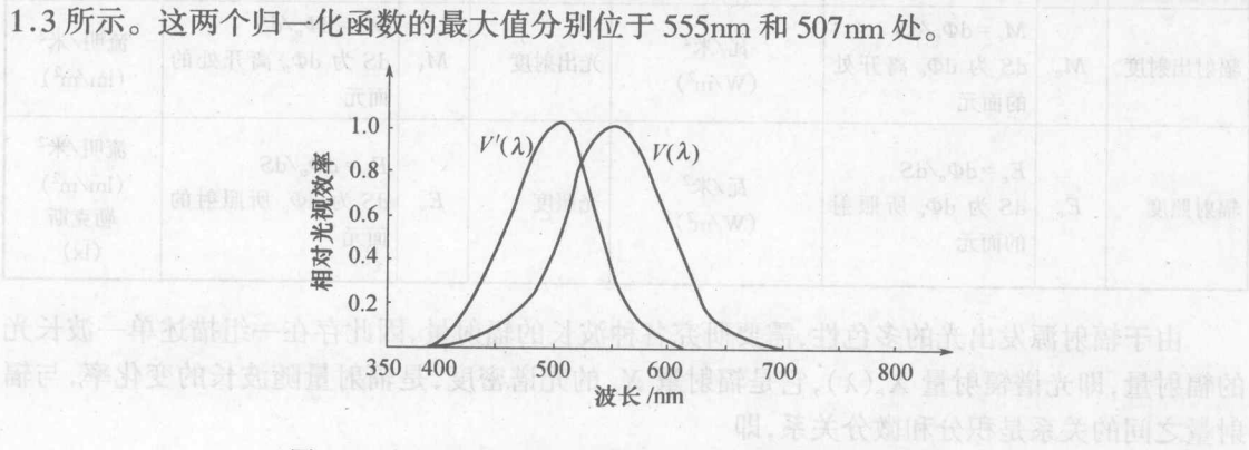
图 1.3 相对光谱光视效率曲线 V(\lambda) (明视) V'(\lambda) (暗视)
