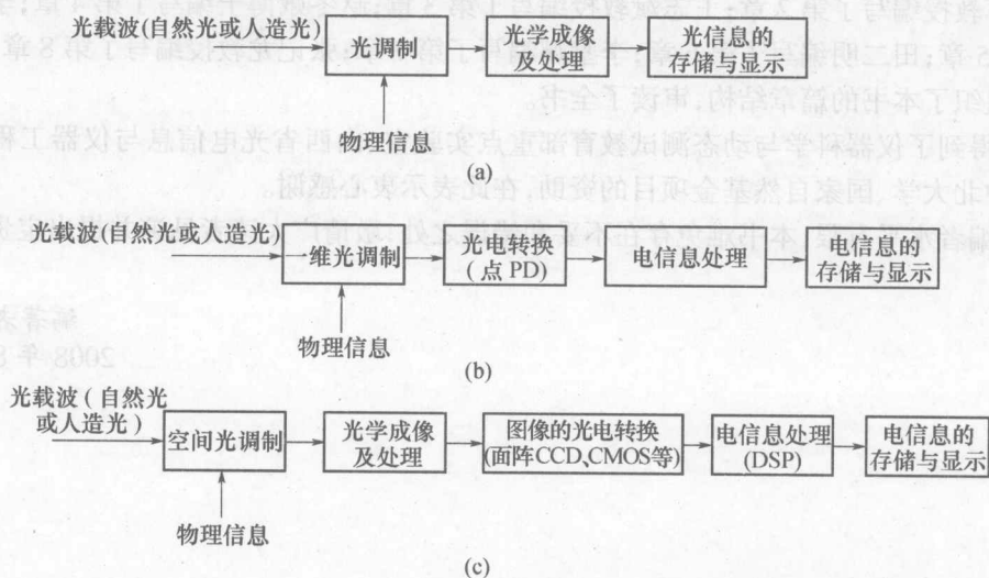
图 1 光电信息系统的分类
