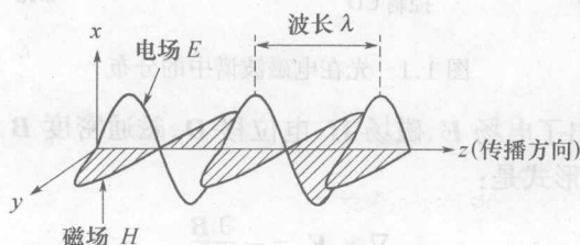
图 1.2 光的传播
