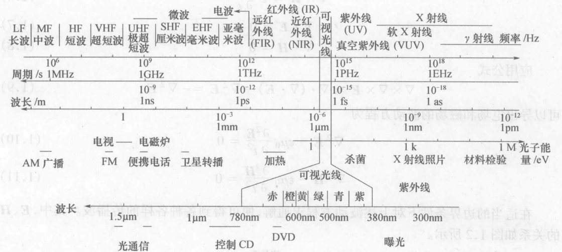
图 1.1 光在电磁波谱中的分布
