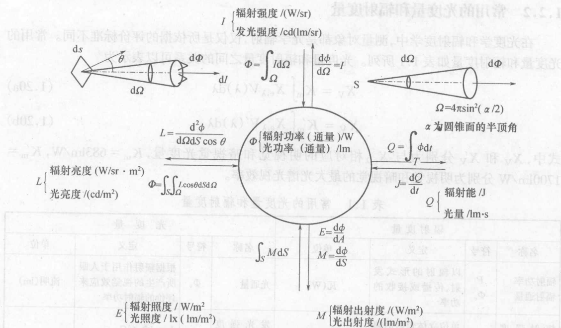
图 1.4 光度量或辐射度量之间的转换关系
