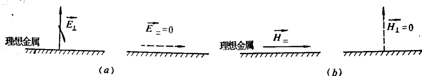
图 1-11 无线电波的边界特性
