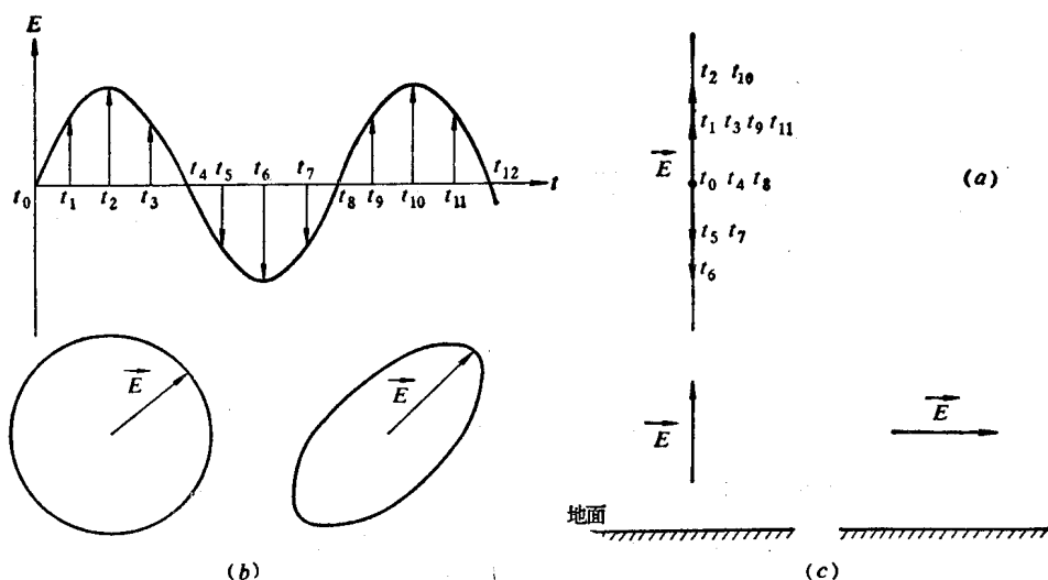
图 1-10 无线电波的极化特性
