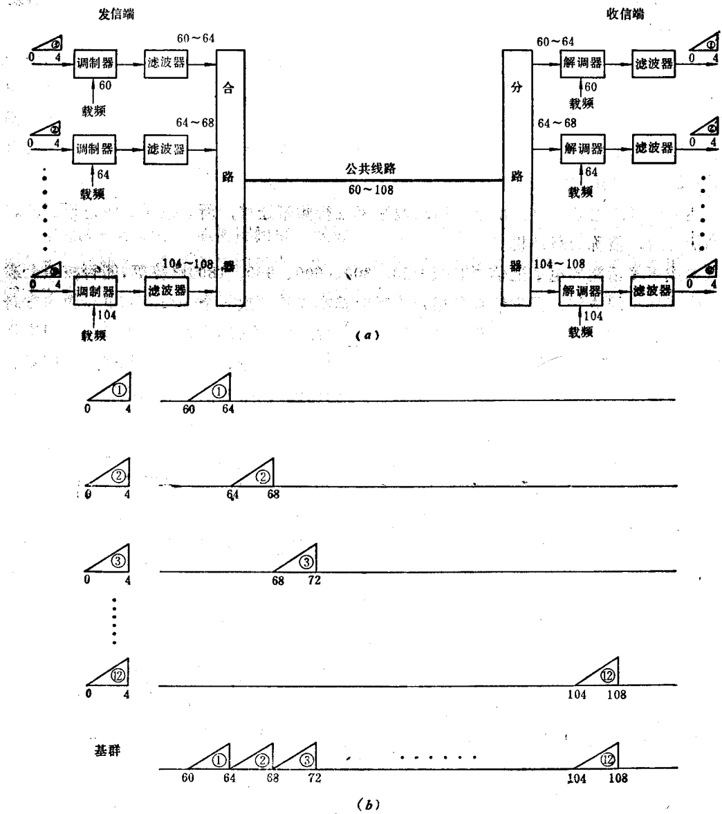
图 1-6 频分制12路电话通信 (a)基本组成; (b)频带迁移 图中：频率单位为KHz。
