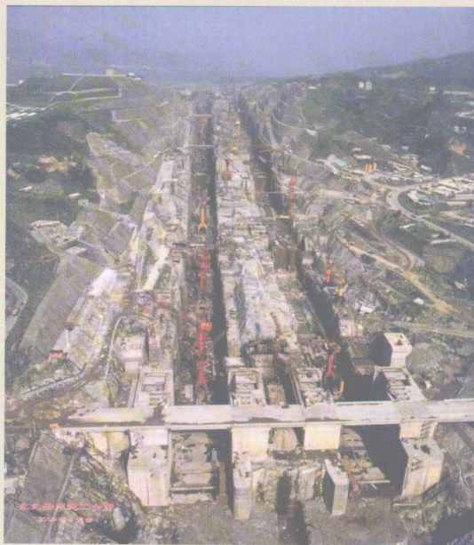
三峡永久船闸雏形
