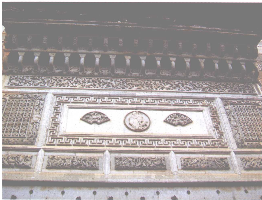
下梅村民居构造
