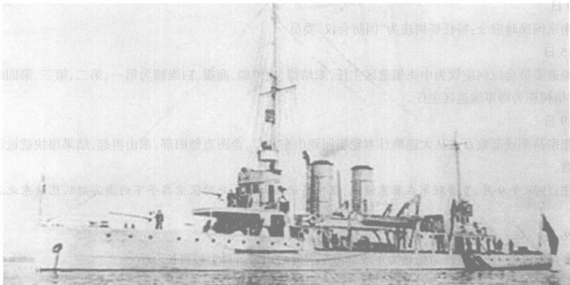
“咸宁”号炮舰于 1929 年初完成时的官方照片
