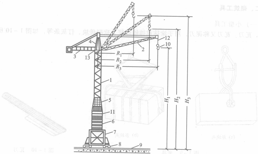
图 1-7 行走式塔吊
