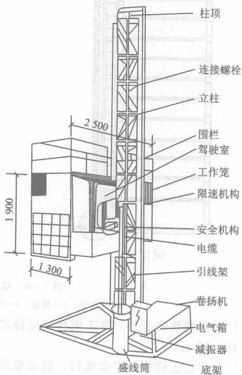
图 1-5 单笼式施工电梯
