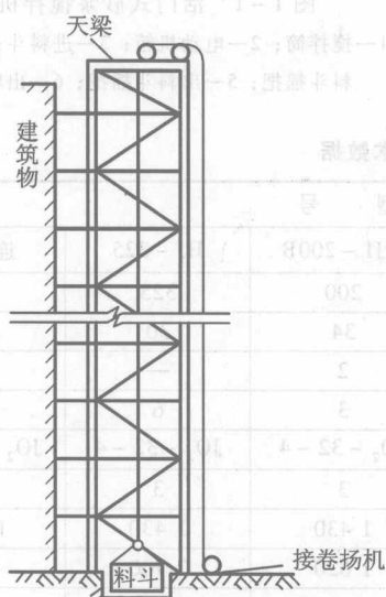
图 1-2 井字架
