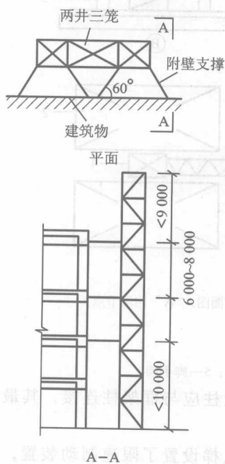
图 1-4 两井三笼井字架的附壁形式
