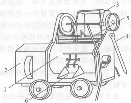
图 1-1 活门式砂浆搅拌机
