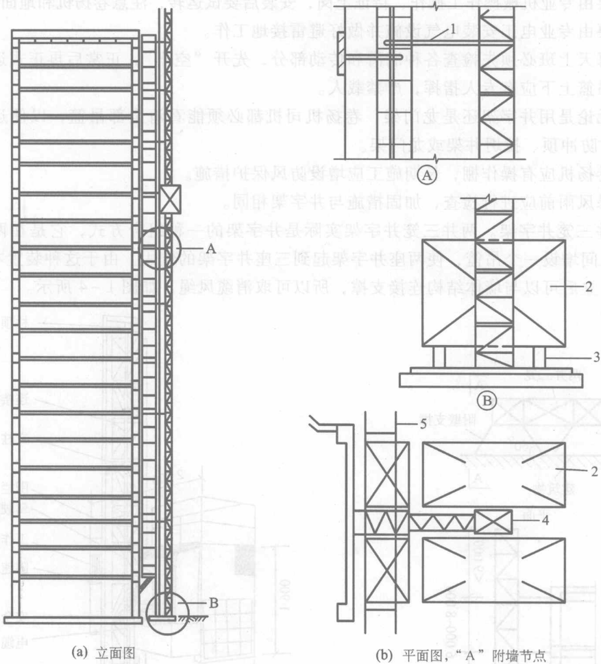
图 1-6 双笼式施工电梯
