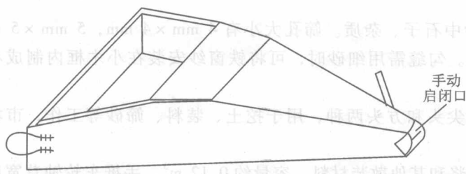
图 1-23 料斗
