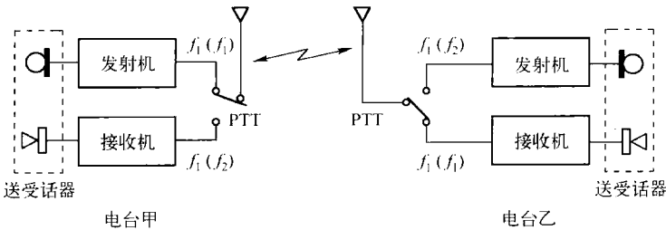
图 1-1 单工通信
