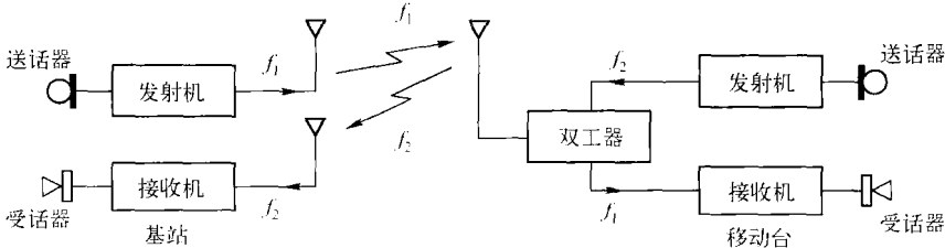
图 1-2 双工通信
