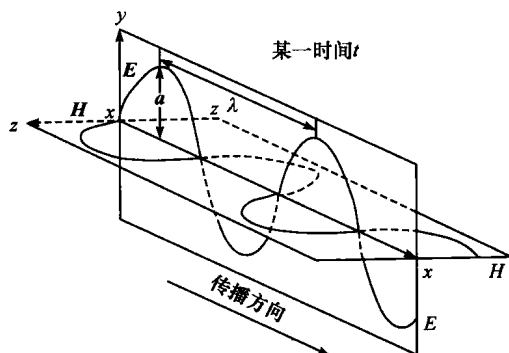
图 1-1 平面电磁波传播示意图
