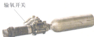
应急氧气筒
