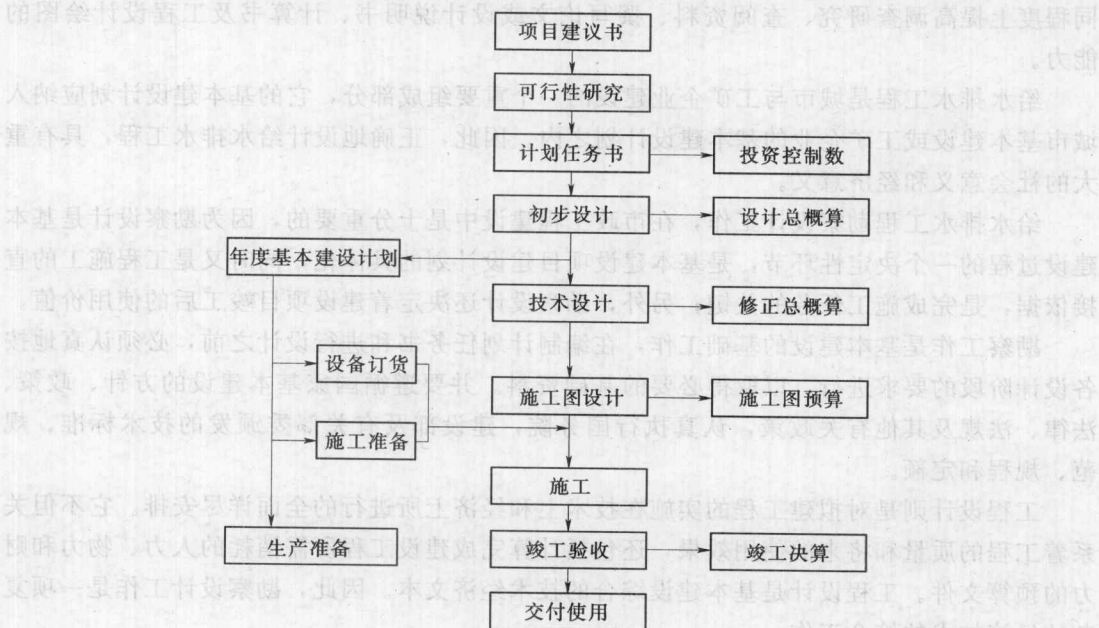
图 1-1 基本建设程序示意图
