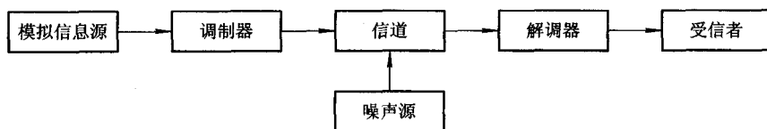
图 1-4 模拟通信系统模型
