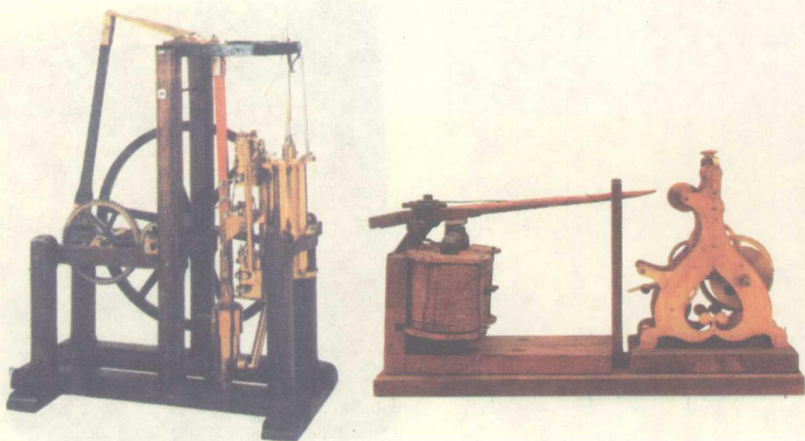
彩图 36 瓦特发明的蒸汽机(1784 年)和莫尔斯码接收机(1849 年)
