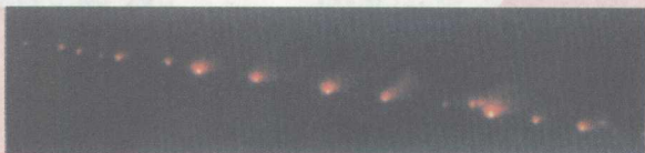
彩图 13 苏梅克-列维 9 号彗星分裂成 20 多块以每秒 60 千米的速度撞击木星,其中最大的碎块直径 4 千米,撞击产生的蘑菇云比地球还大
