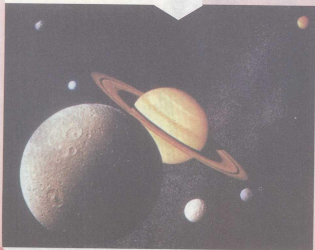
彩图 15 这是旅行者 1 号拍摄的土星系图像,土卫 4 在前,土卫 6 在右上
