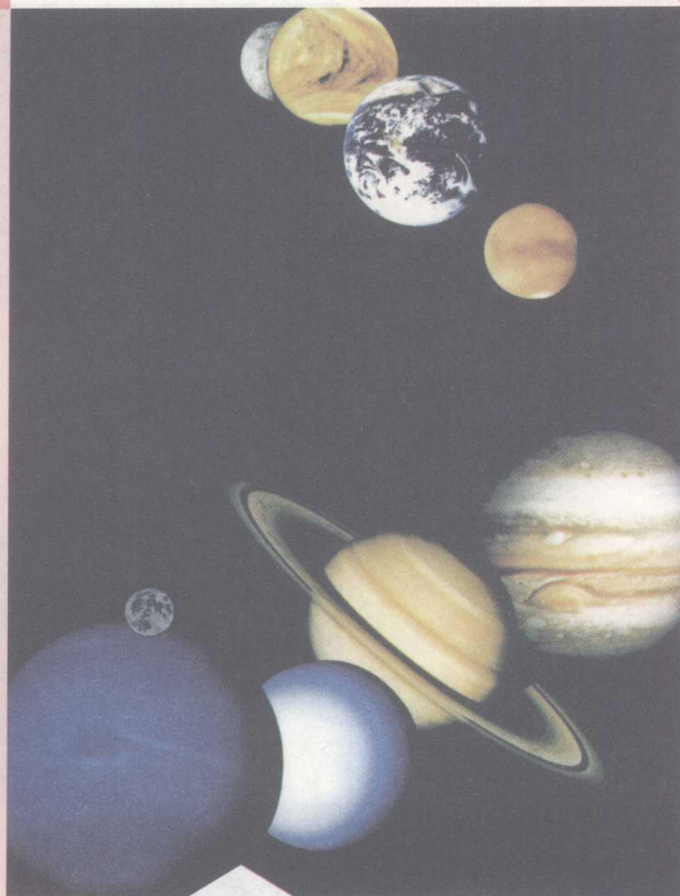
彩图 20 九大行星合影
