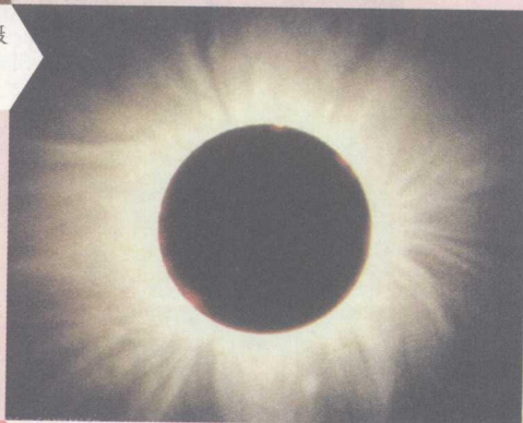
彩图 3 这是在一次全日食时拍摄的日冕照片,其范围达几百万公里
