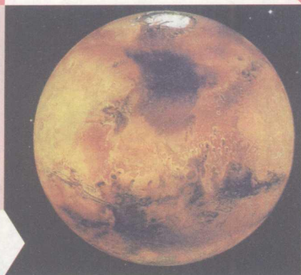
彩图9 火星上的奥林匹斯山是太阳系中最高的山，高度是地球上珠穆朗玛峰的三倍
