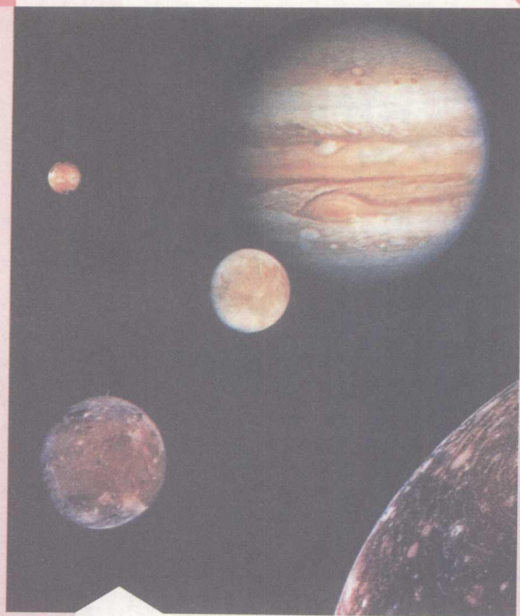
彩图 14 木星和它的 4 颗伽利略卫星,右下为木卫四,左下为木卫三,左上为木卫一,中间为木卫二
