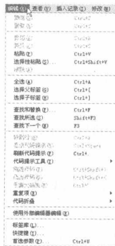
图 1-17 “编辑”菜单
