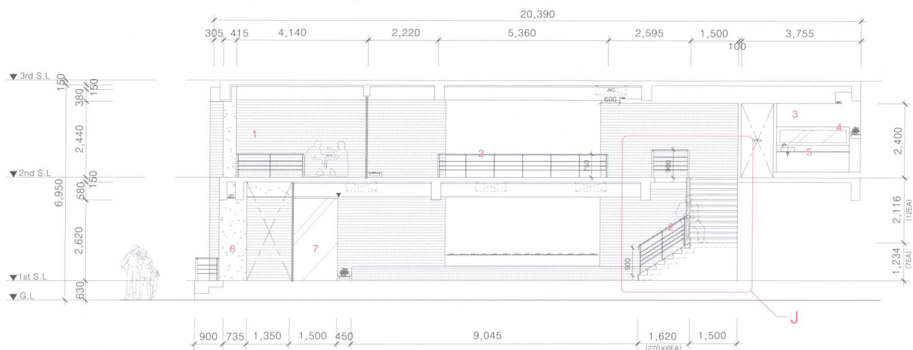
室内剖面图C
