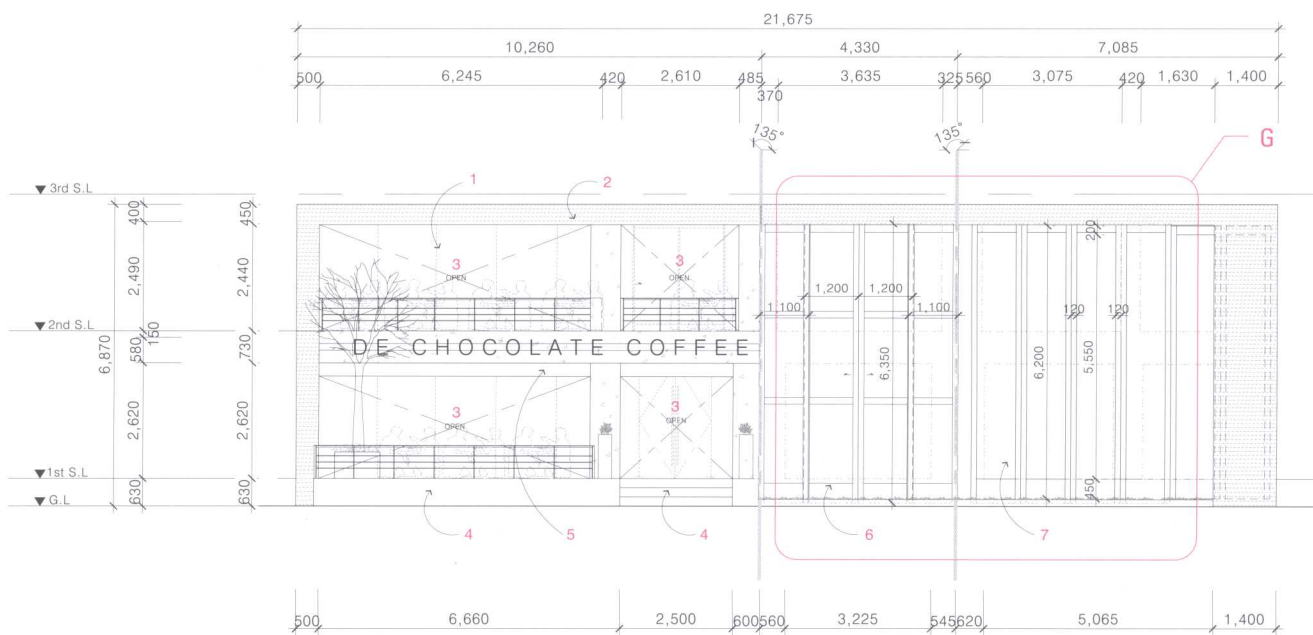
店面立面图 A
