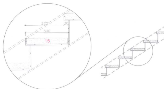
楼梯竖向详图L
