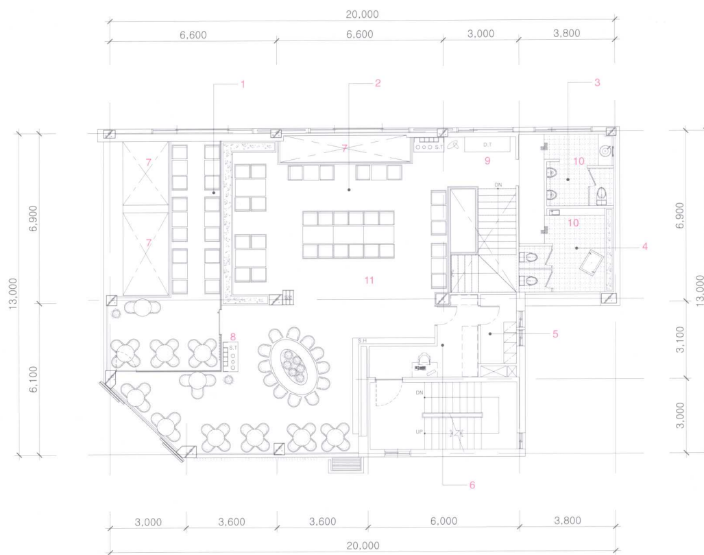
2层平面图
