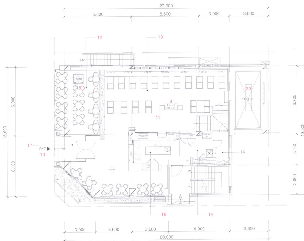
1层平面图
