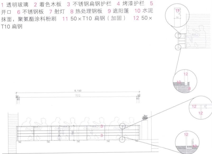
1层进口处露台护栏详图I
