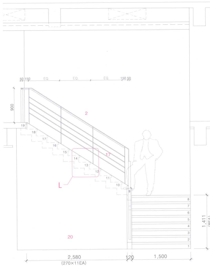
楼梯立面图 J
