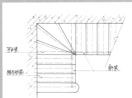
踏步板细部
