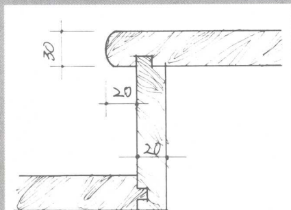
踏步板细部
