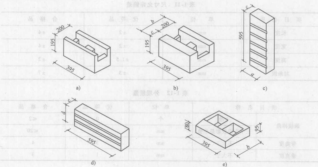
图 1-1 砌模外形及尺寸
