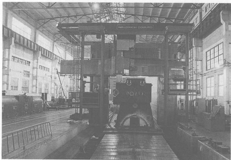
船用柴油机厂从德国引进的重型数控龙门铣床
