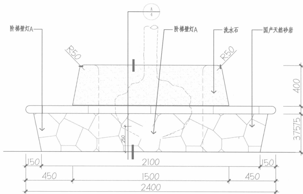
座椅立面图
