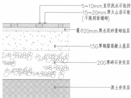
B 铺地剖面图
