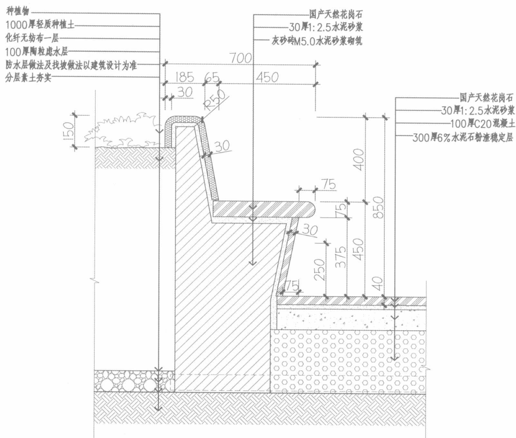
A 座椅剖面图
