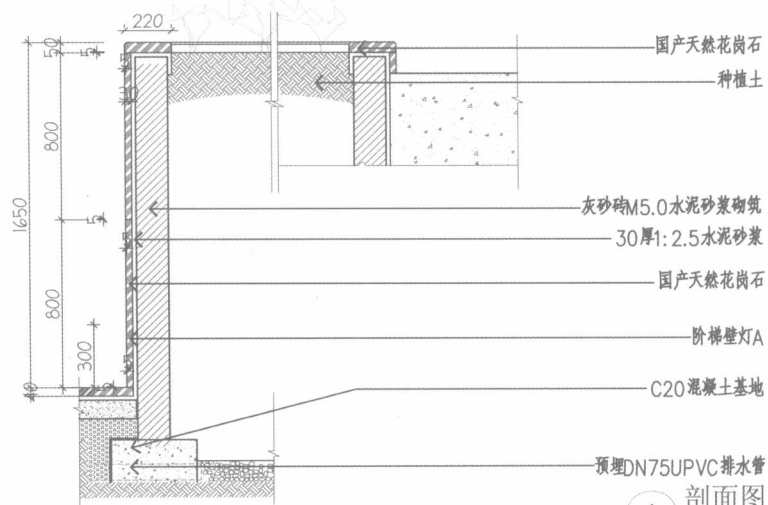
剖面图
