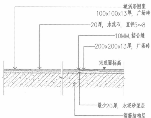
A 铺地剖面图
