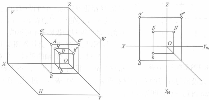
图 1-22 两点的相对位置
