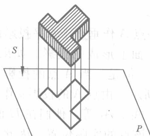
图 1-3 正投影法
