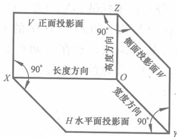
图 1-13 三面投影体系
