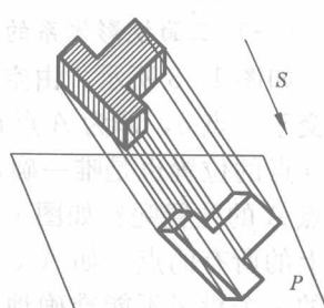
图 1-4 斜投影法
