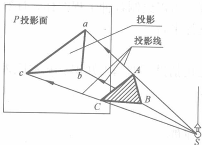
图 1-1 中心投影法
