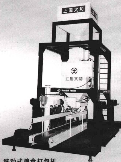
移动式粮食打包机
