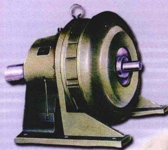
BW型单级摆线针轮减速机
