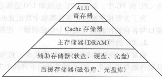
图 1.4 存储器的层次结构
