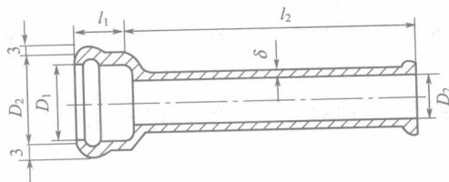
图 1-2 排水铸铁管
