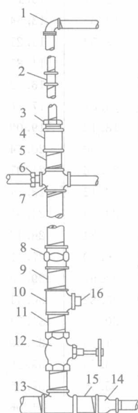
图 1-1 管螺纹连接管件
