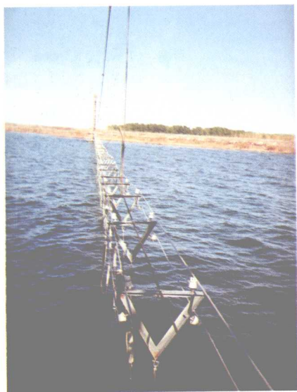
月亮泡水库电栏栅
