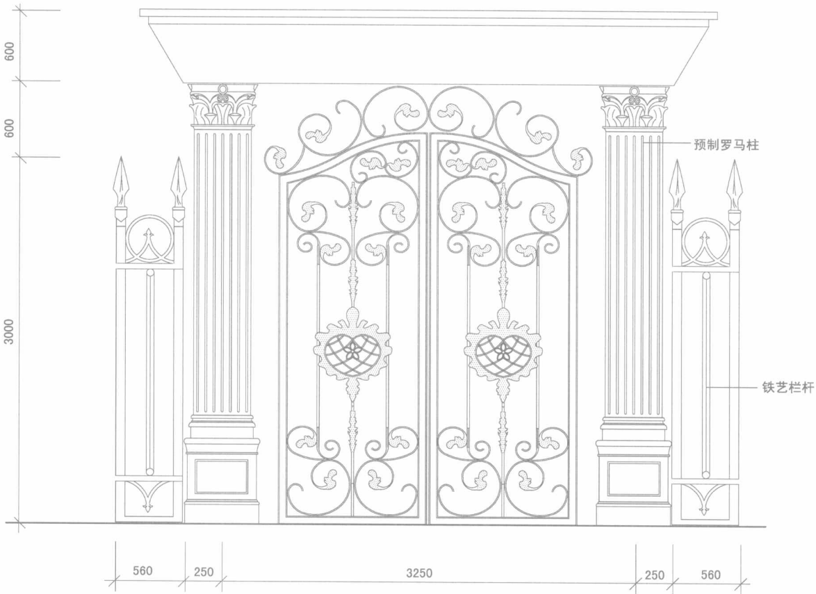
大门立面
