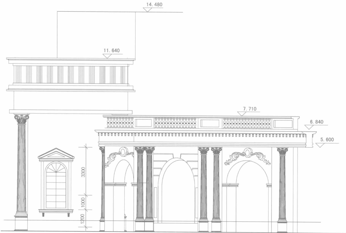
2-D~1-12 轴立面
