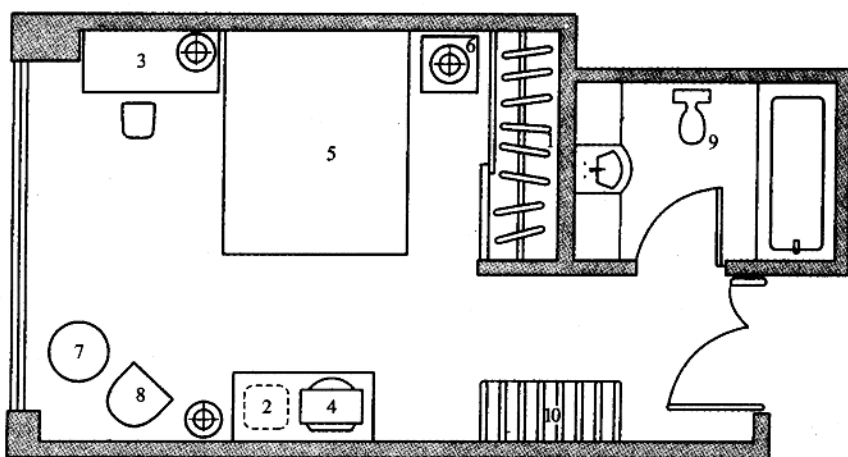
图 1-1 大床间客房平面图
