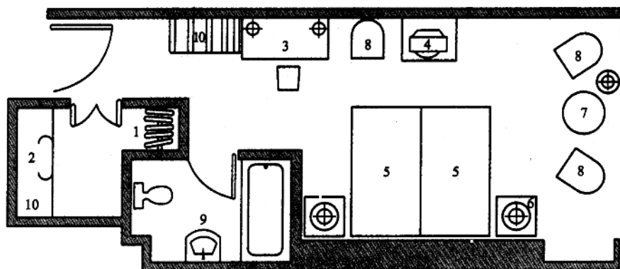
图 1-2 标准间客房平面图
