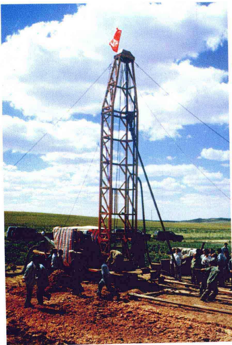
◀ “881” 井灌工程
