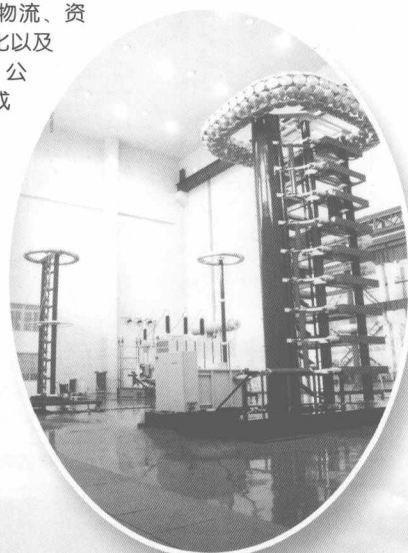
大型变压器实验大厅
