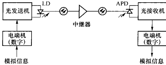
图 1-1 数字光纤通信系统
