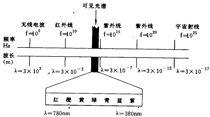
图 2-1 可见光光谱的范围
