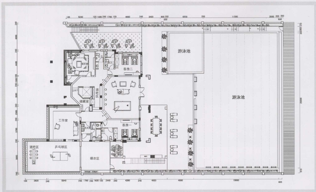
一层平面布置图
