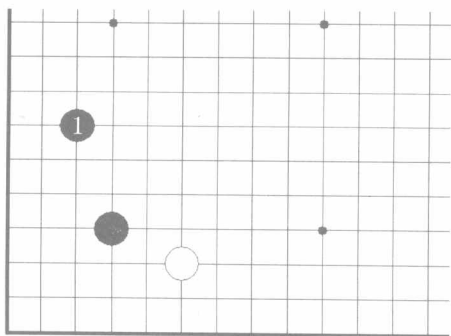
图 1 星定式 17
