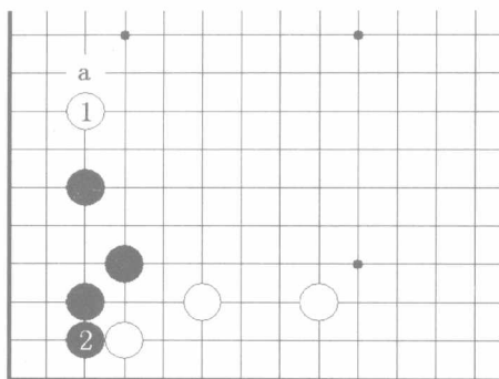
图3 星定式3
