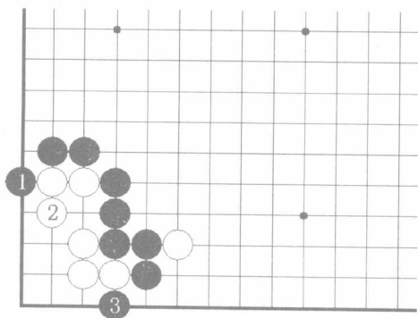
图11 星定式11
