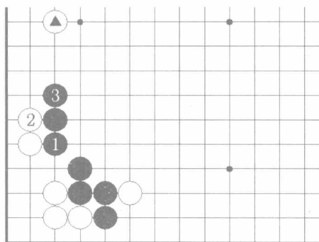
图 13 星定式 13
