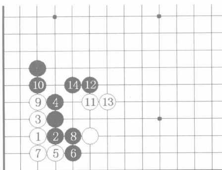
图2 星定式 18
