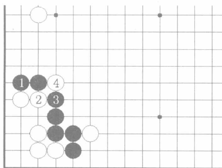
图 14 星定式 14
