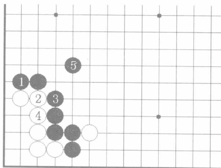
图10 星定式10
