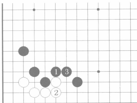
图6 星定式6
