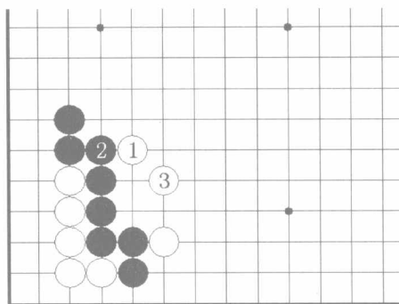
图3 星定式 19
