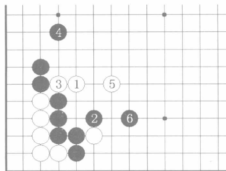
图4 星定式 20
