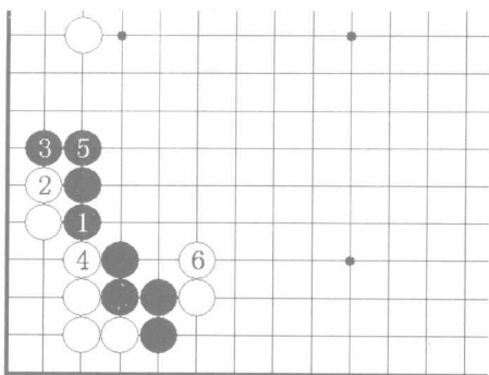
图 15 星定式 15
