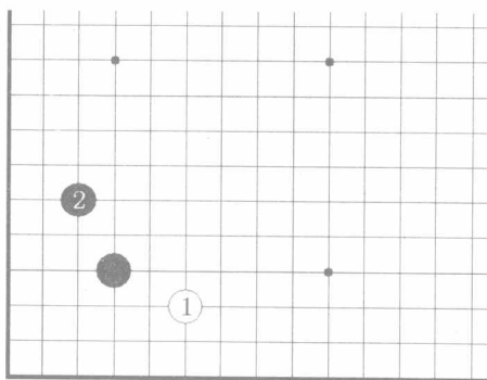
图1 星定式1
