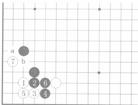
图9 星定式9
