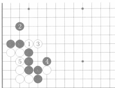
图 12 星定式 12
