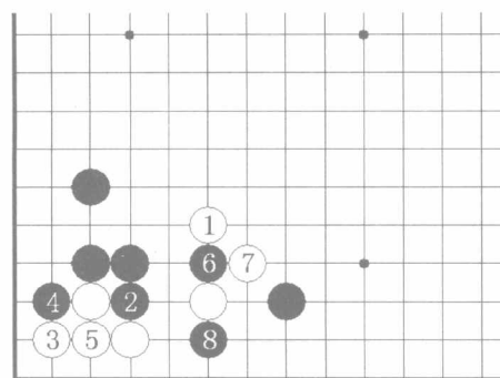
图8 星定式8
