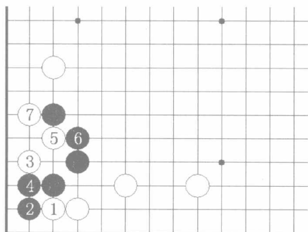
图4 星定式4
