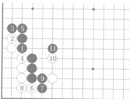
图7 星定式 23
