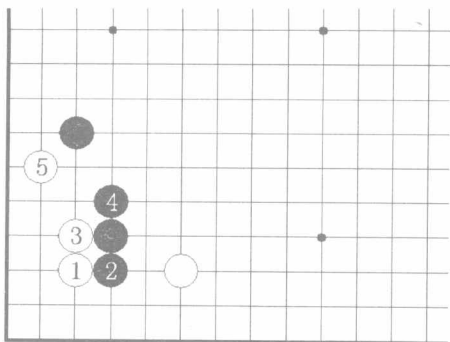
图5 星定式 21
