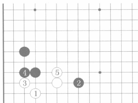
图7 星定式7
