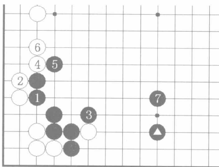
图 16 星定式 16
