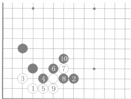
图5 星定式5
