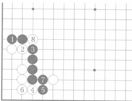
图6 星定式 22
