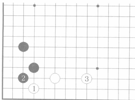
图2 星定式2
