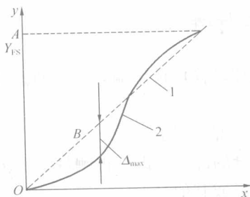
图 2-2 非线性误差说明
