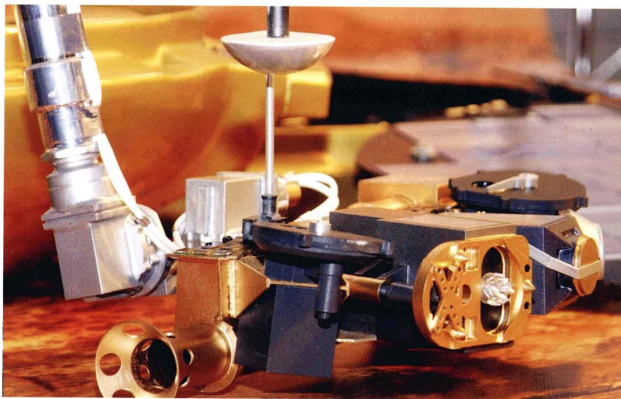
由香港 12 位科研人员研制并成功登陆火星的“岩芯取样器”
