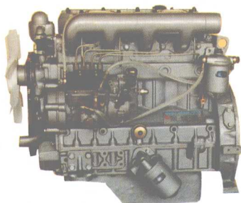
TY495 柴油机
